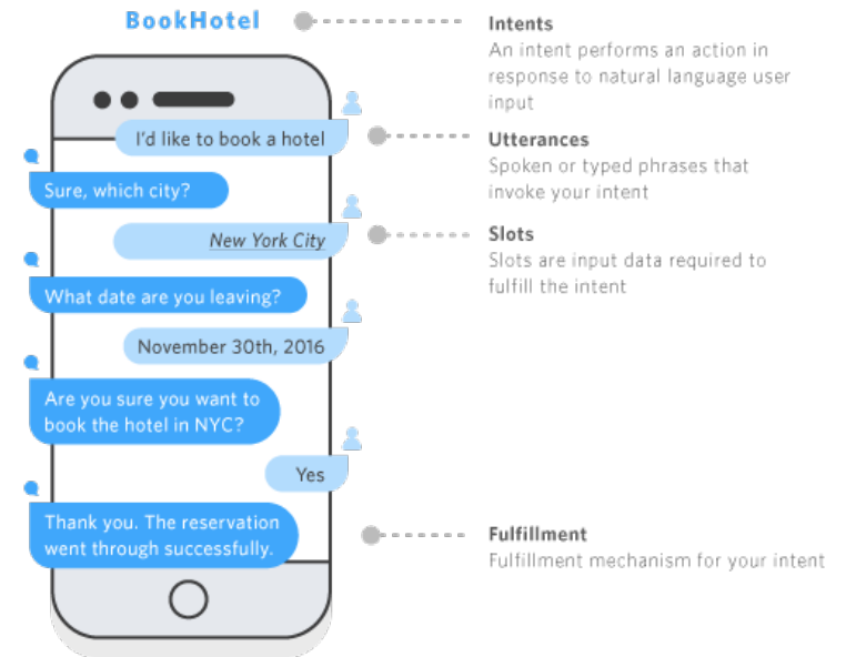
Amazon Lex의 기본 구성 요소 ▶
