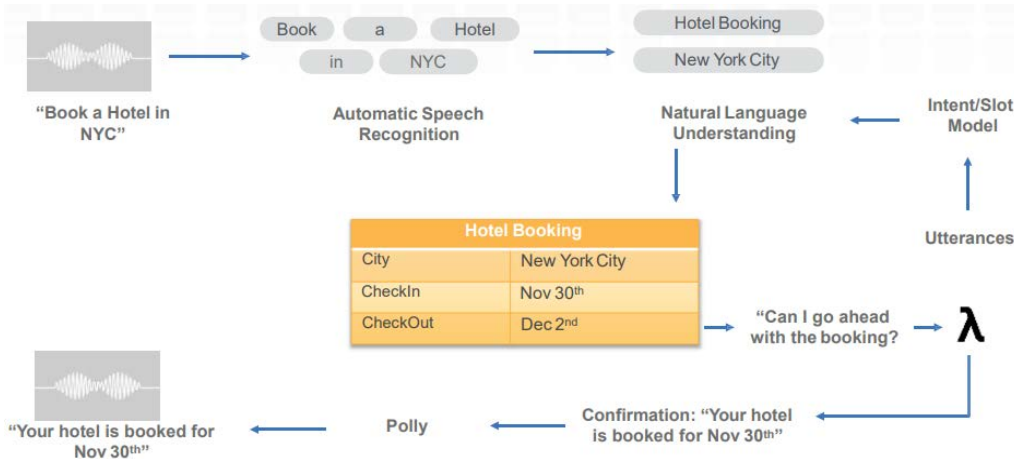
▲ Amazon Lex를 이용한 호텔 예약 시나리오
